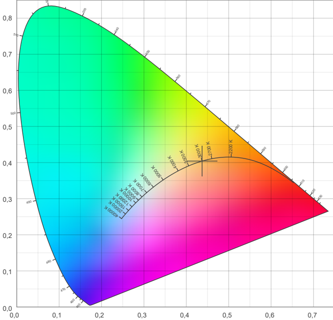
CIE 1931
